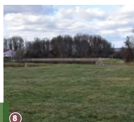
8 Boisement
