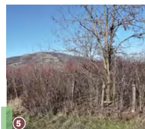
⑤ Pré-bois
