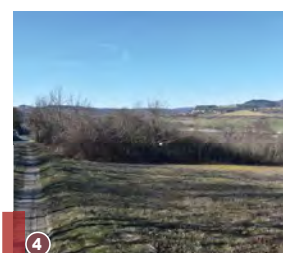
④ Landes
