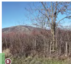
5 Pré-bois
